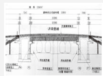
大島陸橋側面図
